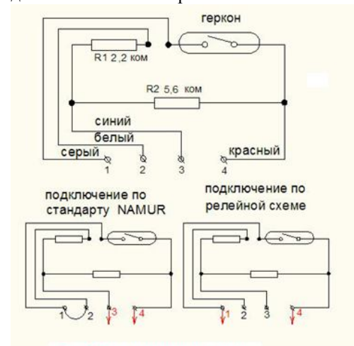
Рис.3 Схема импульсного выхода
